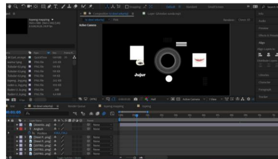
Gambar 16. Animasi Background
